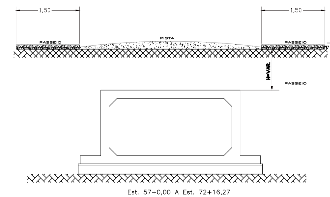
GALERIA FECHADA SEM ESCALA
