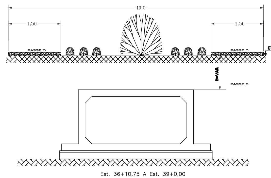
GALERIA FECHADA SEM ESCALA
