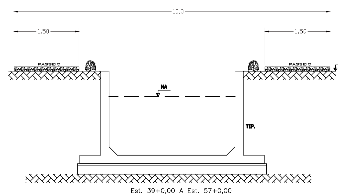
CANAL REVESTIDO SEM ESCALA
