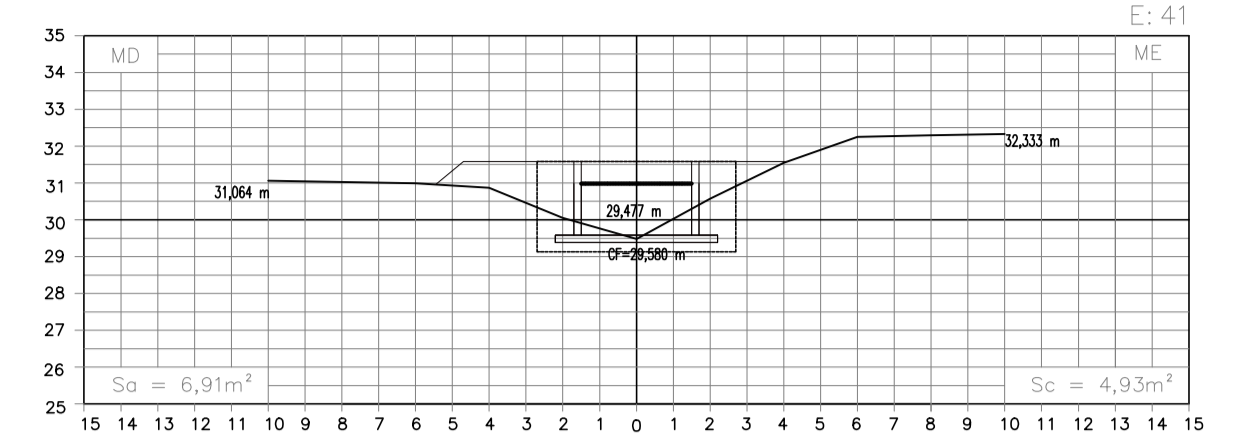
SEÇÕES TRANSVERSAIS ESC.: H=1/200 V=1/200
