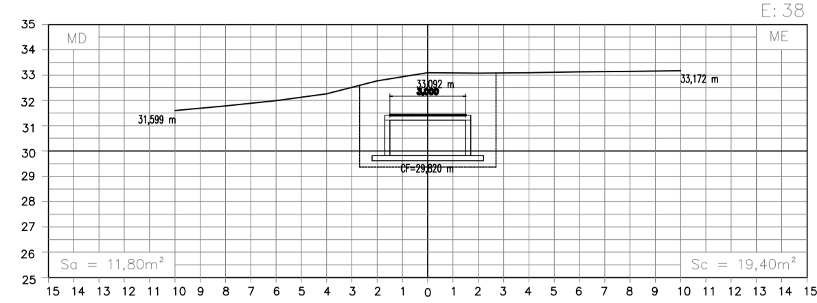
SEÇÕES TRANSVERSAIS ESC.: H=1/200 V=1/200
