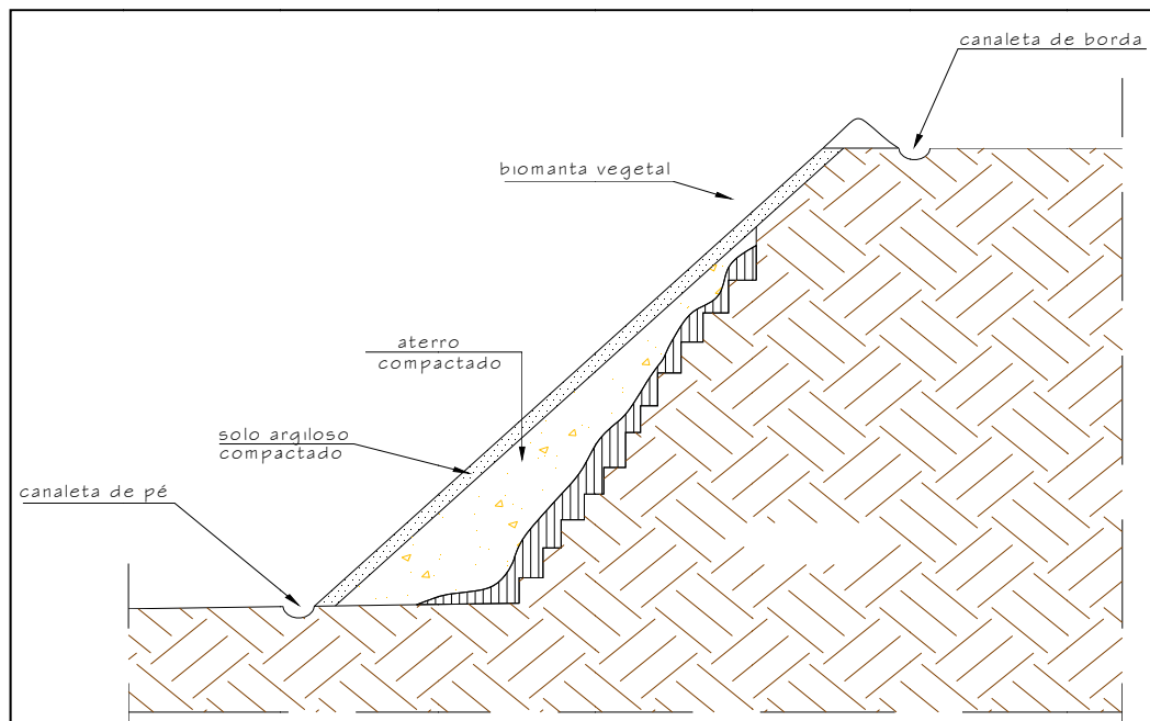
RETALUDAMENTO CONTÍNUO
