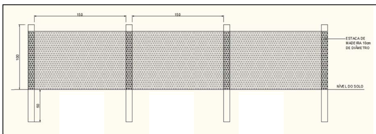
PROJETO-TIPO DE FIXAÇÃO DA BARREIRA DE SILTAGEM.
