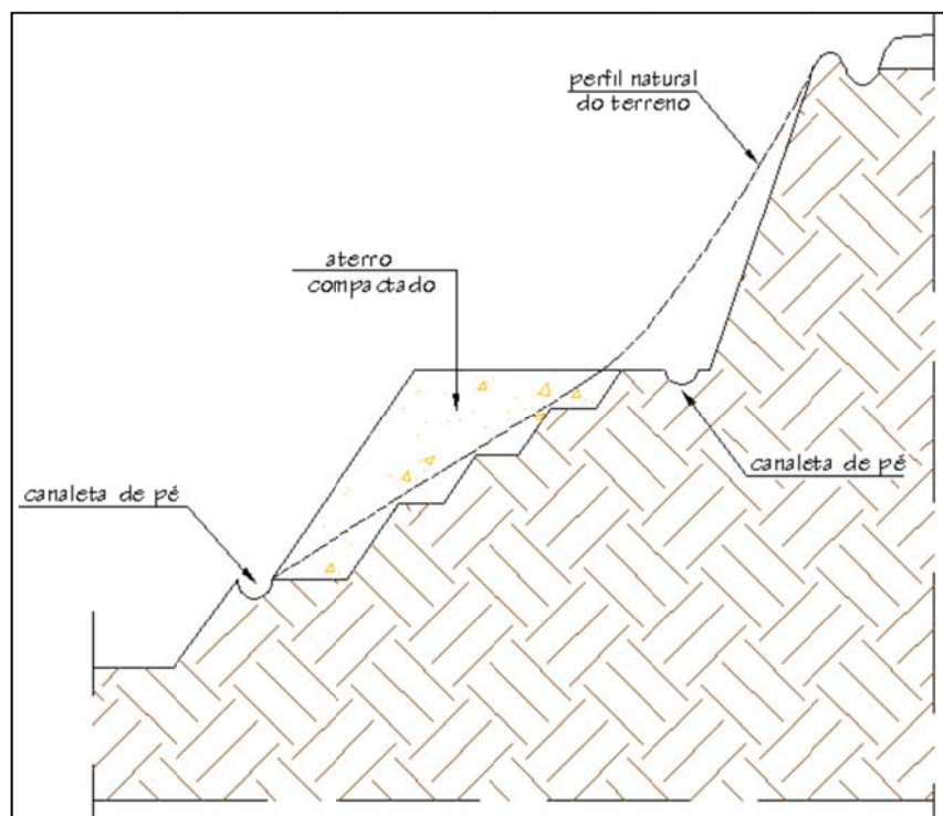
RETALUDAMENTO ESCALONADO
