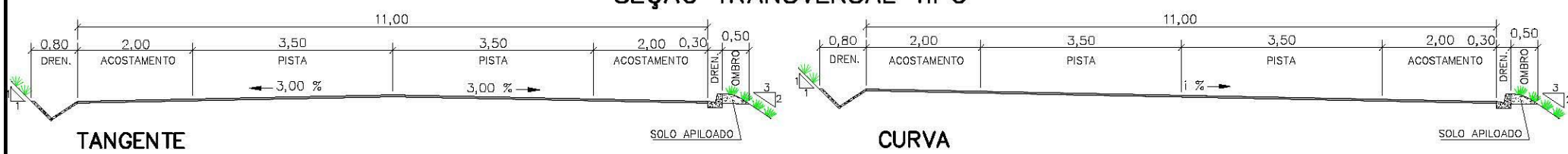
RODOVIA SEÇÃO TRANSVERSAL TIPO
