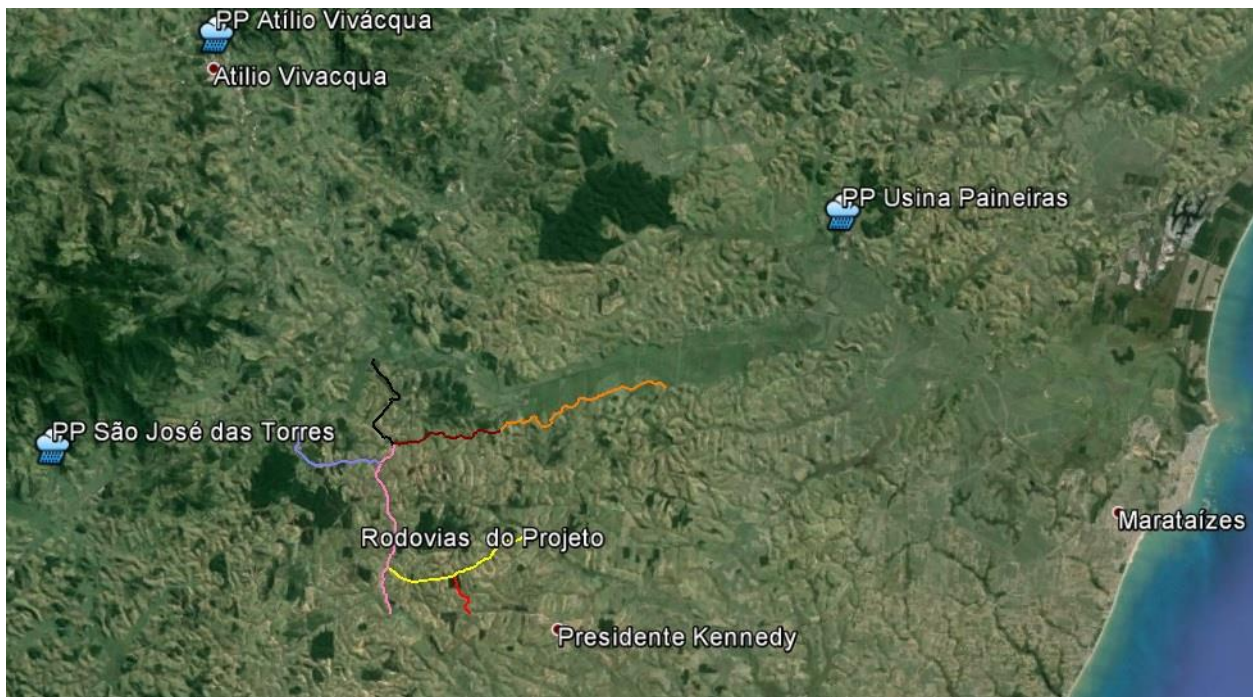
Figura 3.7.1 Localização das Estações Pluviométricas
