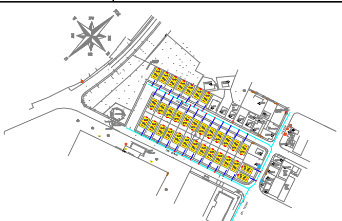
SISTEMA DE ADUÇÃO DE ÁGUA
