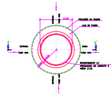
PLANTA BAIXA ESCL: 1:20
