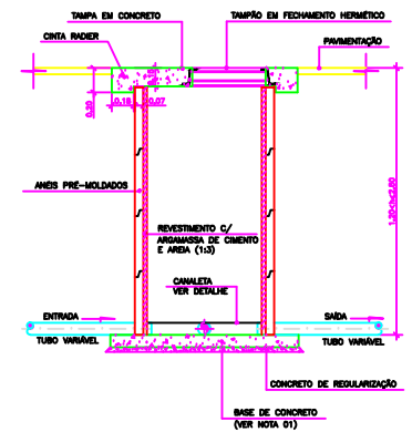
CORTE AA' ESCL: 1:20
