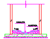
DETALHE DA CANALETA 1/ ESC.
