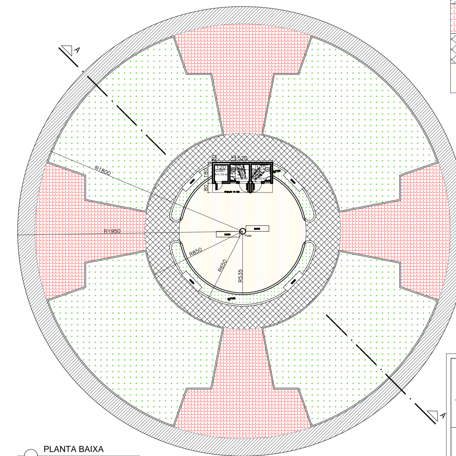
PLANTA BAIXA Esc 1:200
